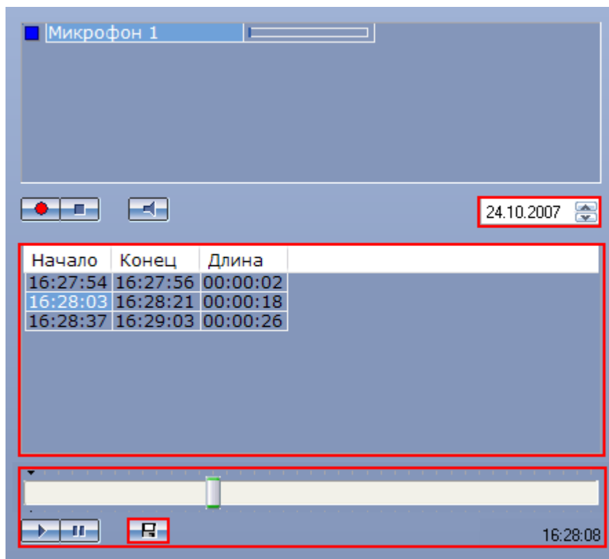
Рис. 4.4-19. Элементы интерфейса Аудиопроеигрывателя для экспорта аудиозаписей, созданных по акустопуску или команде Оператора
