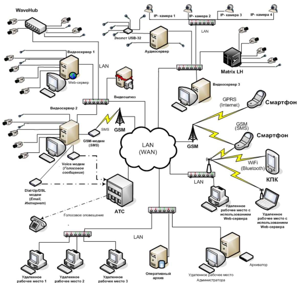
Рис. 3.3-1. Универсализированная структурная схема цифровой системы видеонаблюдения и аудиоконтроля на базе комплекса «Интеллект ГПН»
