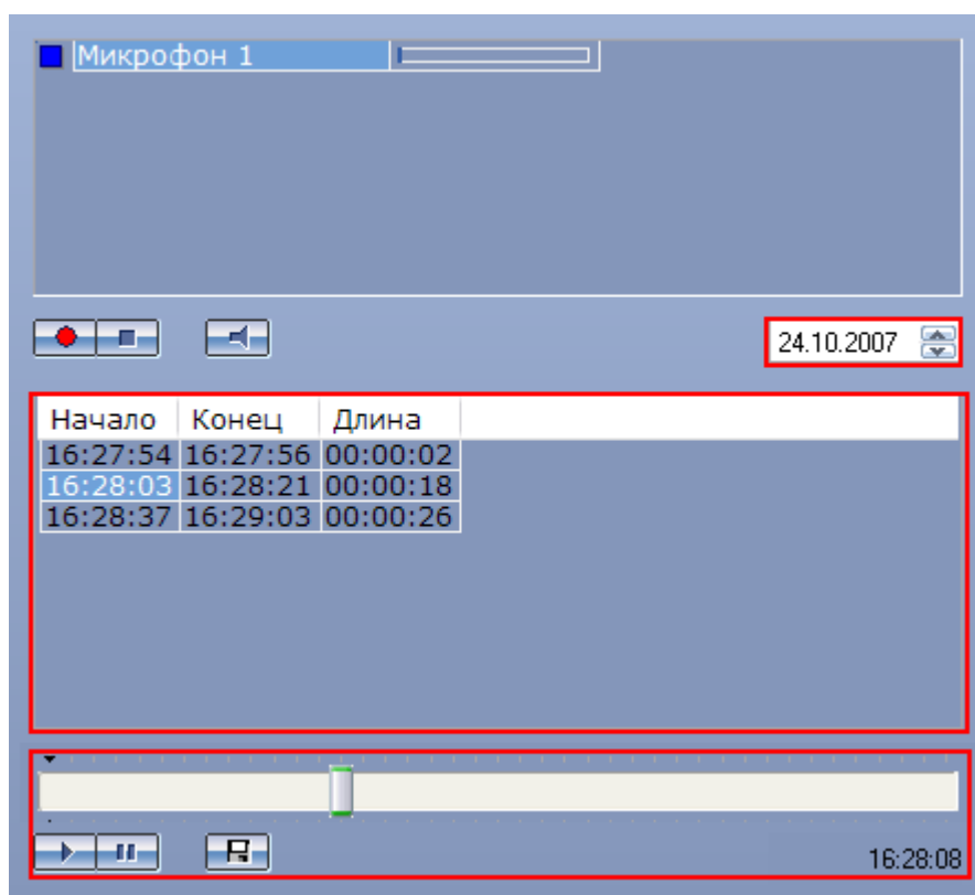
Рис. 4.4-14. Элементы интерфейса Аудиопроеигрывателя для воспроизведения записей
