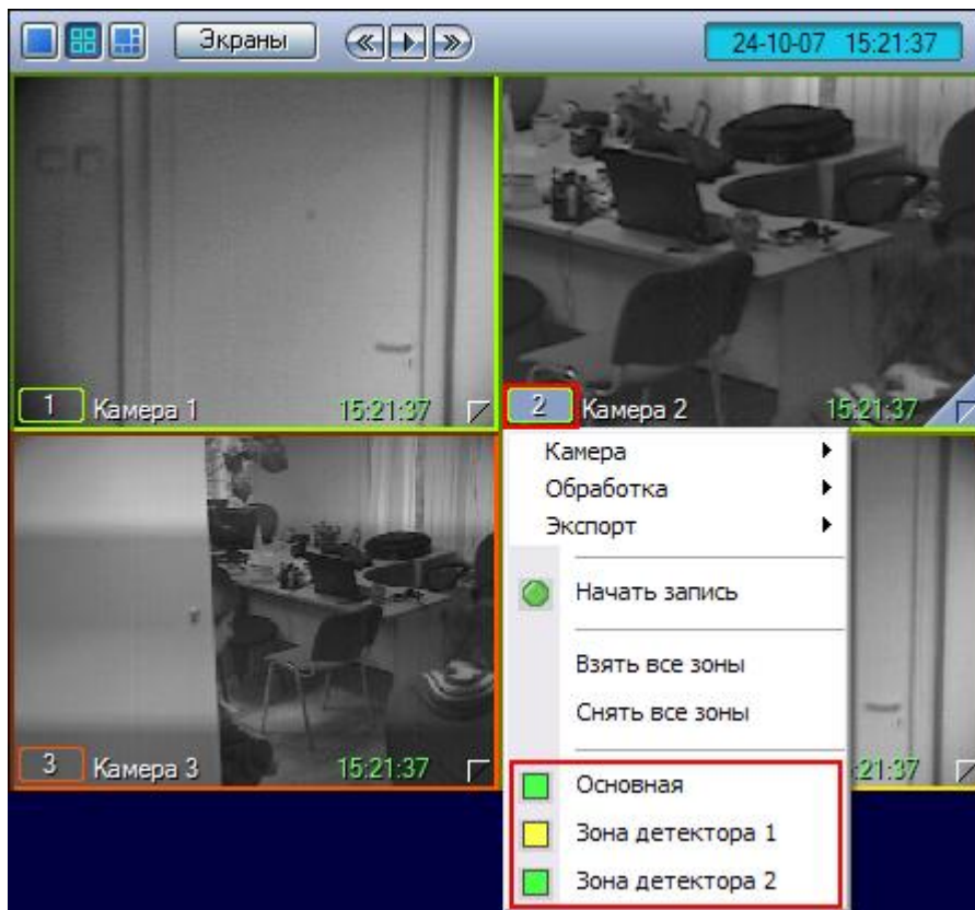
Рис. 4.3-12. Снятие видеочамеры с охраны по дополнительным зонам детекторов
