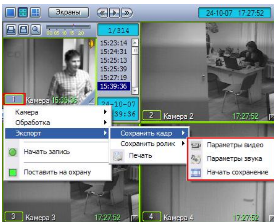
Рис. 4.3-68. Доступ к функции экспорта фрагмента видеозаписи
