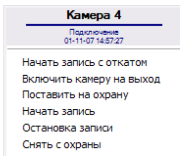
Рис. 4.2-19. Функциональное меню объекта типа «Камера»
